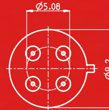
T039 4Pin
