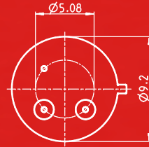
T039 3Pin
