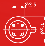
T018 4Pin
